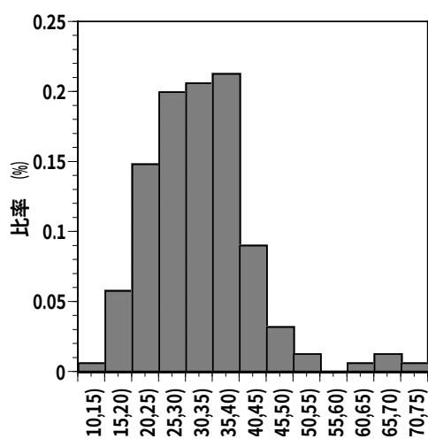
図 3-11 主な土壌特性の確率分布 (ヒストグラム)
