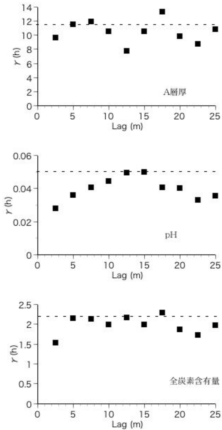
図 4-17(2) 区画 B における主な土壌特性に関するセミバリオグラム
