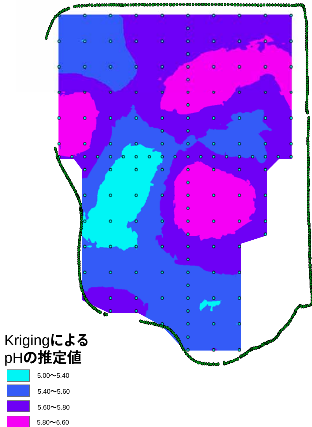
図 5-19 Kriging によって求めた pH の空間分布に対する領域区分
