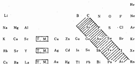
周期律表上の金属と非金属元素の分布図
