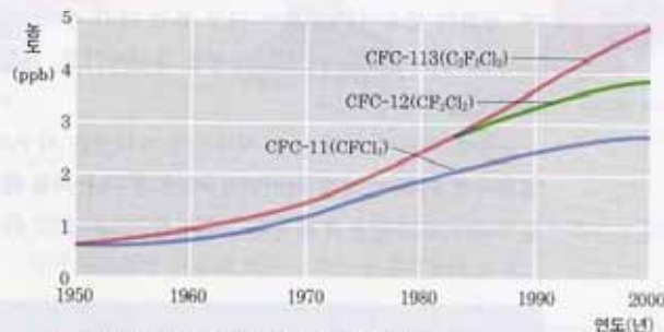
▲ 대기 중에 축적된 염화플루오르화탄소 양의 변화
