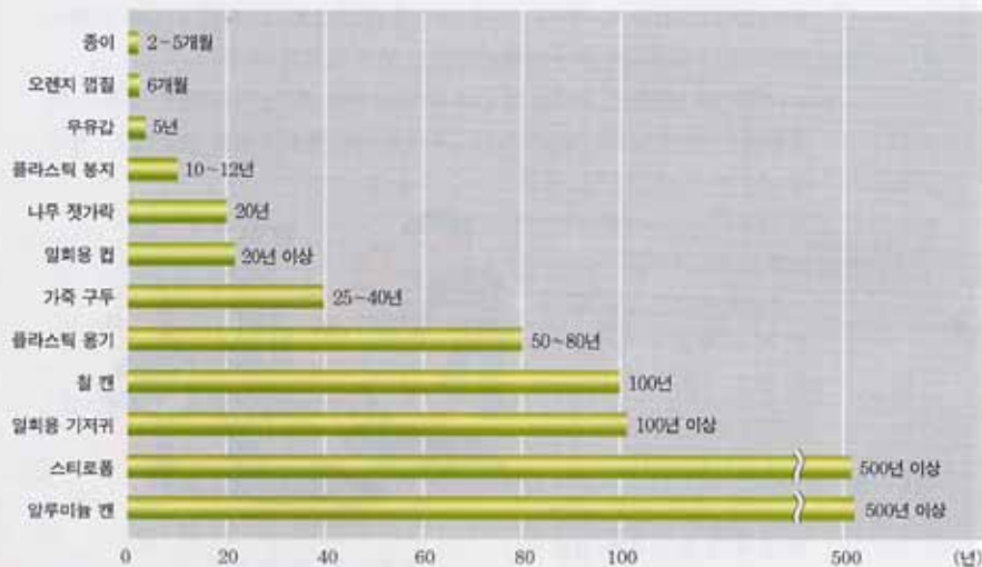
▲ 생활 폐기물이 분해되는 데에 소요되는 기간
