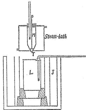
Fig. 4. Calorimeter apparatus.
