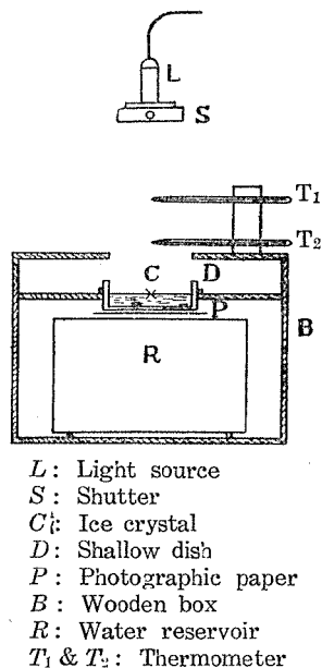
Fig. 1. Apparatus
