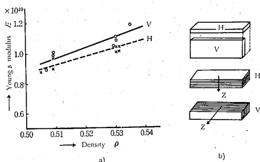
Fig. 26. a) b). Anisotropy of Peter snow; Sample Nos. 23-30, 81-86.
