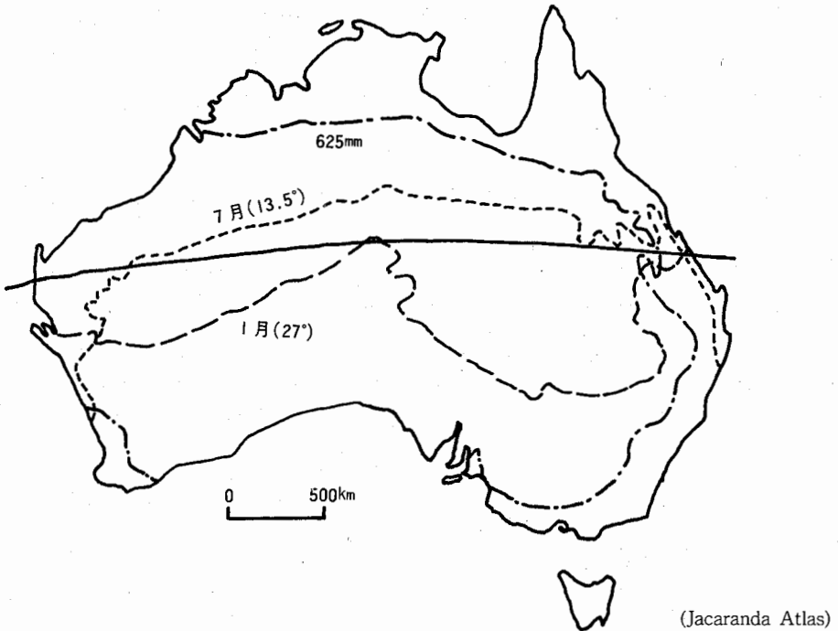
図2 気温と降水量
