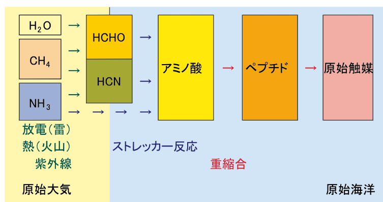
図8：化学進化の古典的シナリオ
