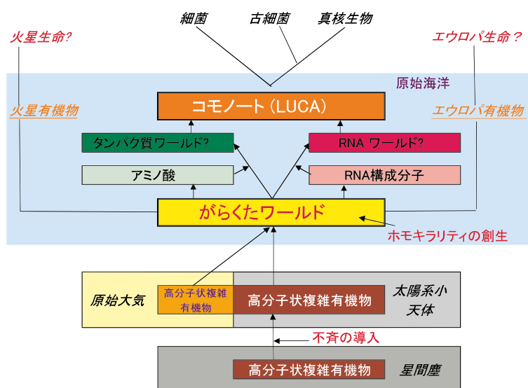
図9：化学進化の新たなシナリオ
