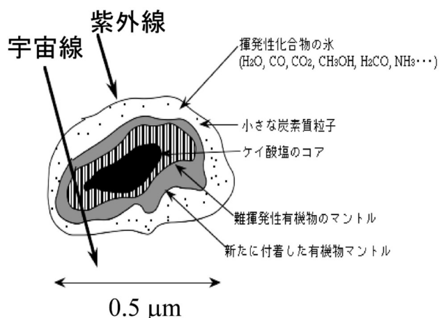
図1: 星間塵アイスマントル中での有機物の生成
