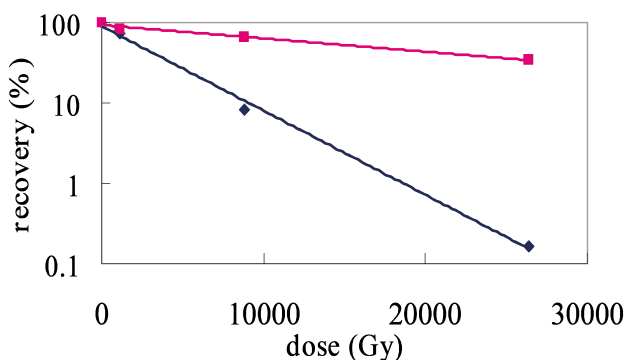
図 5：グリシンと複雑有機物中の結合型グリシンの重粒子線に対する安定性
