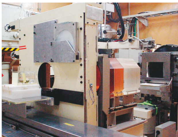
図3：メタン・アンモニア・水混合物への高エネルギー炭素線照射
