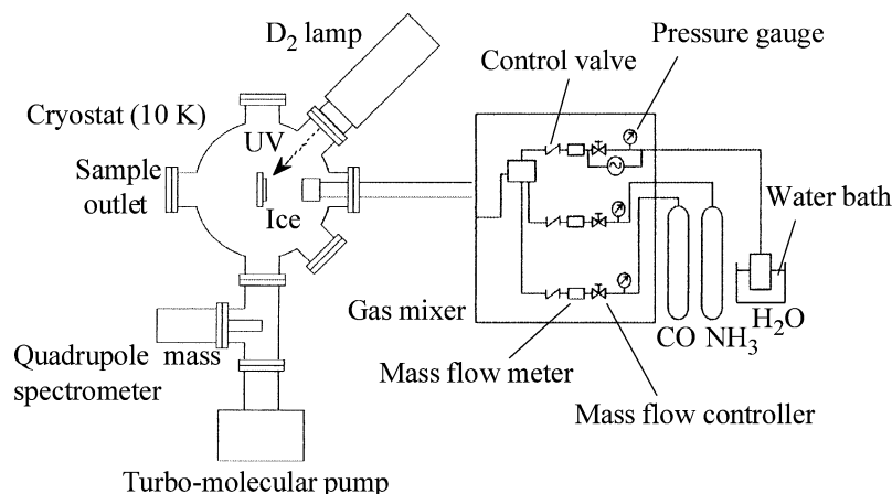
図2：模擬星間塵アISMントルへの紫外線照射実験（文献16より転載）
