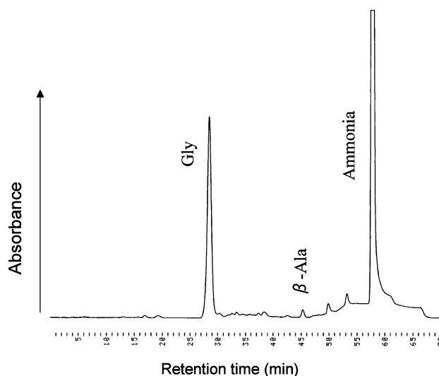
図4：メタノール・アンモニア・水凍結混合物への炭素線照射により生じたアミノ酸（加水分解後）
