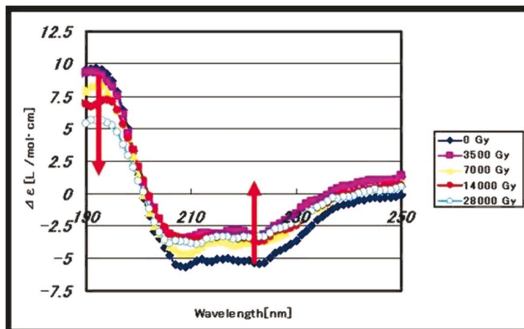
図6：炭素線照射によるヒト血清アルブミンのCDスペクトルの変化 220 nm 付近の負のピークはタンパク質中の \alpha -ヘリックス含量に対応する。
