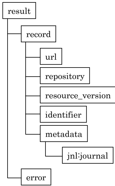
図 3 : ir.xsd
