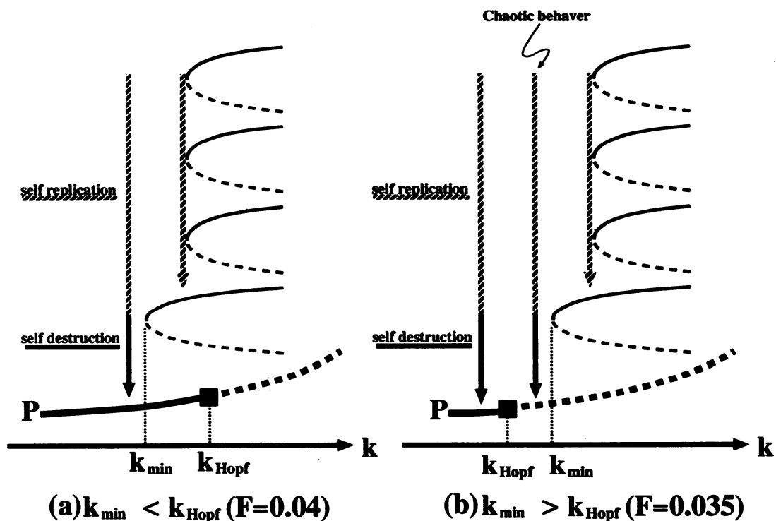
図 6: (a) F = 0.04 . k_{\text{min}} < k_{\text{Hopf}} なので自己複製および自己崩壊はおこるが、 P は安定なので、その後の時間発展はない。(b) F = 0.035 . k_{\text{min}} > k_{\text{Hopf}} が成り立ち、自己崩壊の後、 P が不安定となるパラメータ k をとることができる。そこでは時空カオスが存在する。
