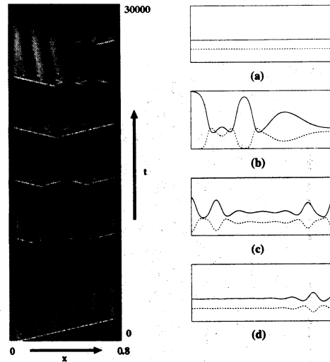
図 1: Gray-Scott モデル (1) における時空カオス ( D_u = 2 \times 10^{-5} , D_v = 10^{-5} , F = 0.035 , k = 0.05632 およびシステムサイズ L = 0.8 ). 右のスナップショットは解がほぼ定数状態 P から出発し、次にいくつかの部分区間で (u, v) = (1, 0) に落ち、そこへまわりから自己複製波が進み、定常パターンがしばらく現れ、そしてそれが自己崩壊して、再び P に戻る一つのサイクルを示している。
