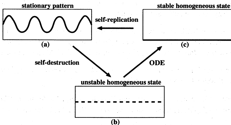
図7: k = k_{min} では \mathbf{R} 上で形式的に定常解、不安定定数解 P 、安定定数解 (u, v) = (1, 0) をめぐるヘテロクリニックサイクルを構成できる。実際の有限区間で観察される時空カオスでは P から (1, 0) へ移るとき、区間全体で一様に行くのではなく(真に (1, 0) へ落ちればそこから軌道は出れない)、必ず自己複製波が生み出される (1, 0) 以外の部分が残っている。実際、上のサイクルはある部分区間に着目すれば観察できる。図1を見よ。
