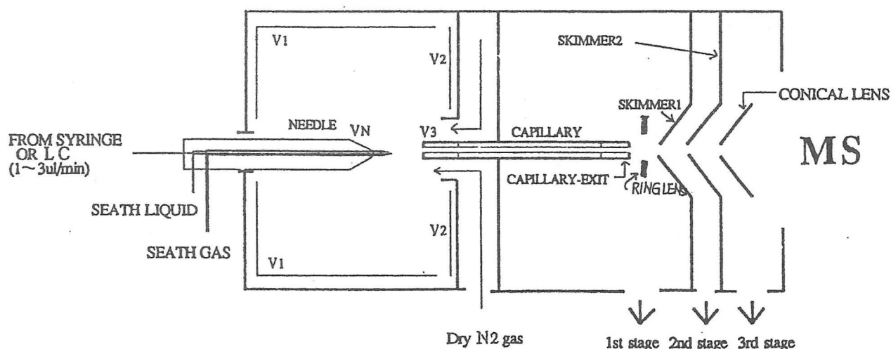
図-1 ESIイオン源の概略図
