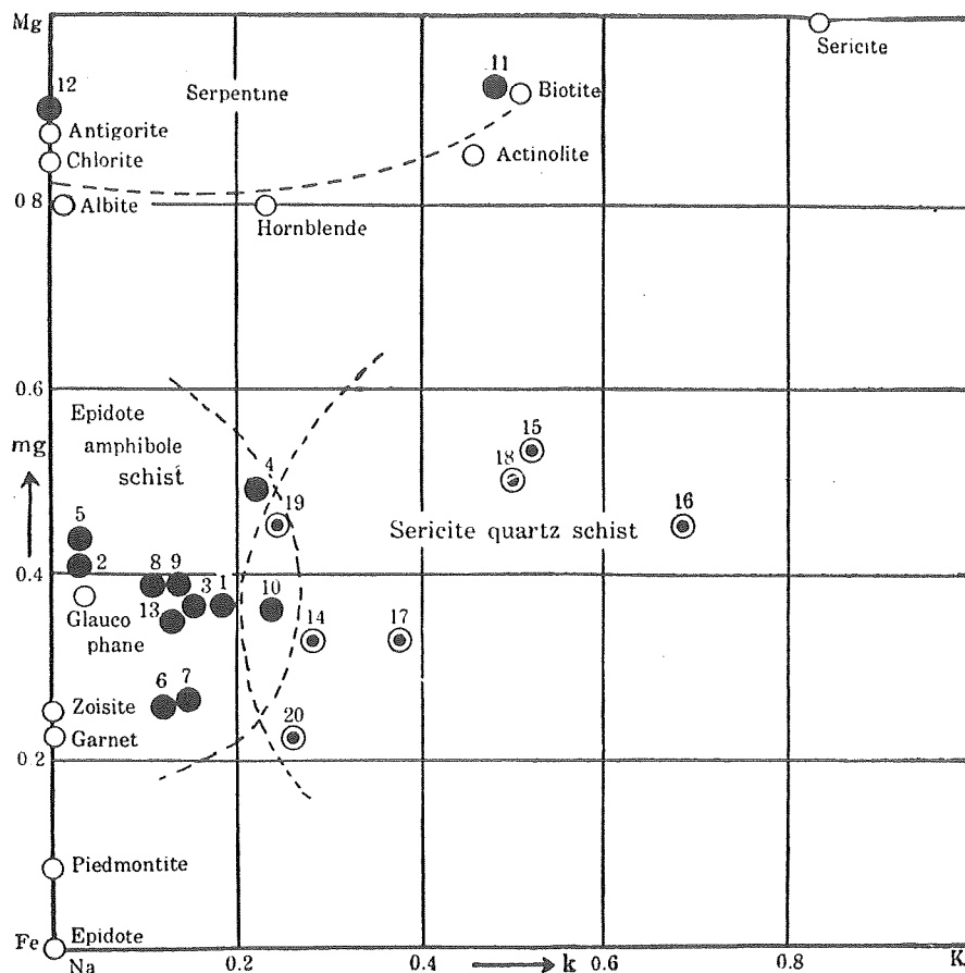
Fig. 7. mg-k-Diagram.
