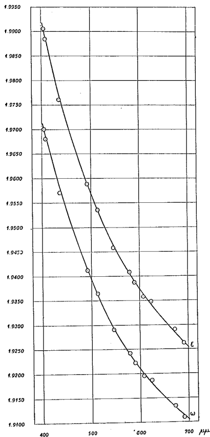
Fig. 4. Lichtbrechungen des braunen Scheelits von Tyûnanmen, Urusan, Korea.
