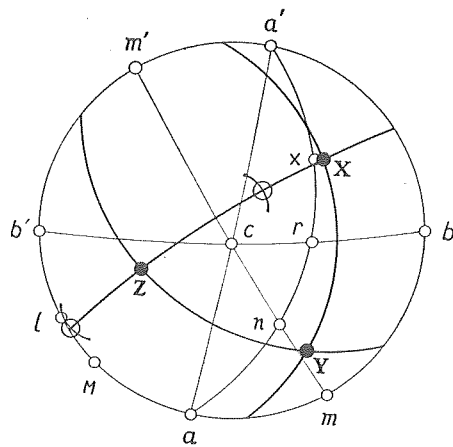
Fig. 2. Stereographische Projektion des Axinites von Toroku mit eingetragenen optischen Oertern.
