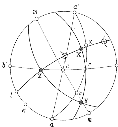
Fig. 1. Stereographische Projektion des Axinites von Obira mit eingetragenen optischen Oertern.
