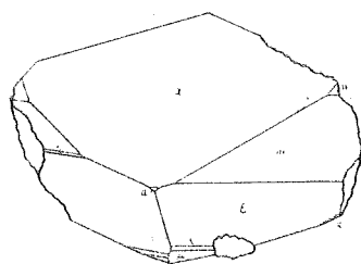
Fig. 4. Crystal I
