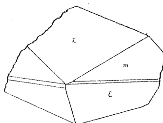
Fig. 7. Crystal V
