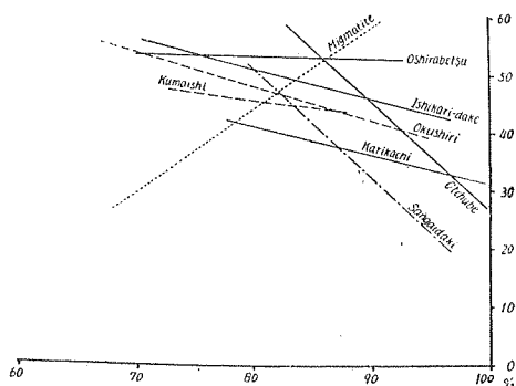
Fig. 4c. Plagioclase
