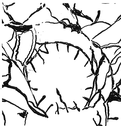
Fig. 6. Thysanophyllum aseptatum DOBROLYUBOVA
