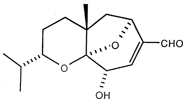
1i
