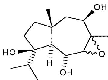
36 [53]
