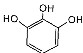
pyrogallol (74)
