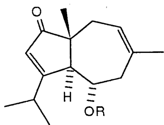
45 R=p-anisate [46]
