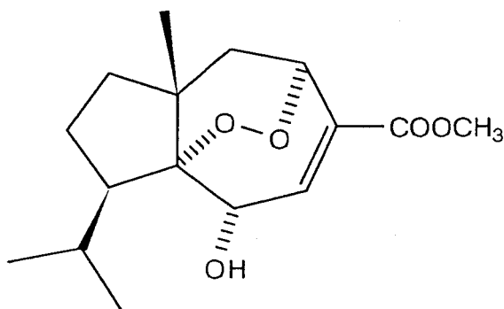
1k
