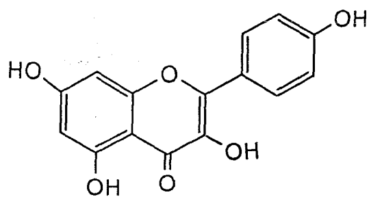
kaempferol (71)
