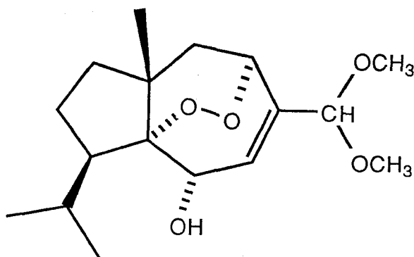
1h
