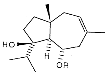
43 R=angelate [44]
