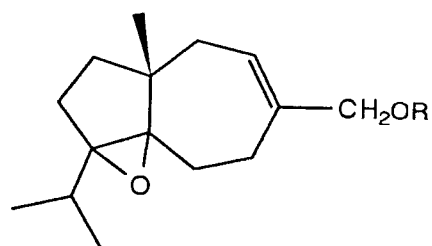
46 R=p-anisate [46]
