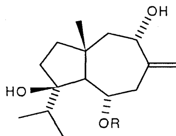
38 R=isovanillate [48]
