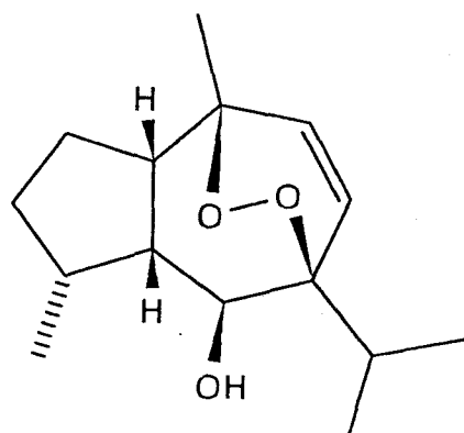
guaia-6,9-diene (79)
