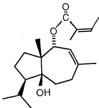
lasidiol (55) angelate
