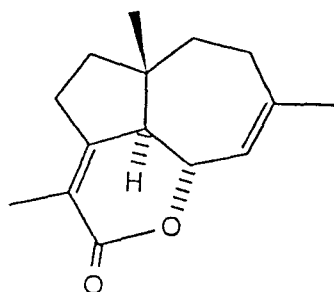
56 [59]
