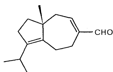
9; daucenaldehyde (RL-A)
