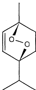
ascaridol (86)
