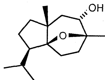
daucol (29)
