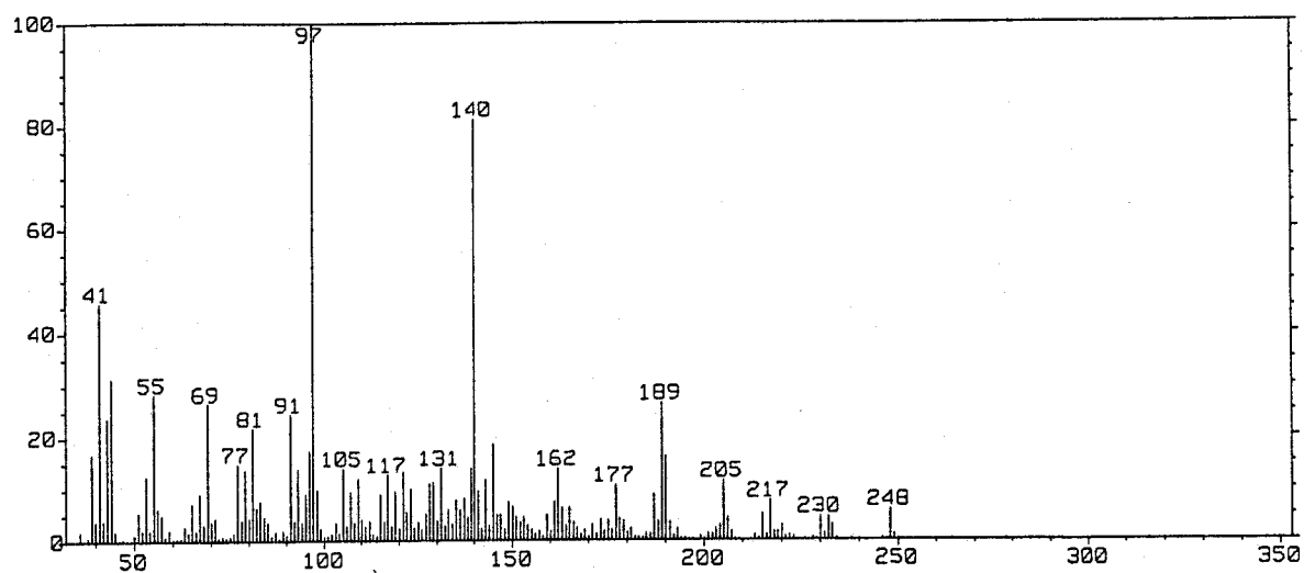
Fig. 3-124 EI-Mass Spectrum of RDA-TU
