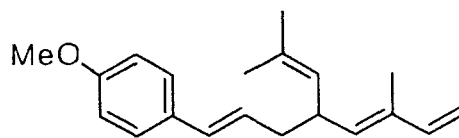
juvocimene I
