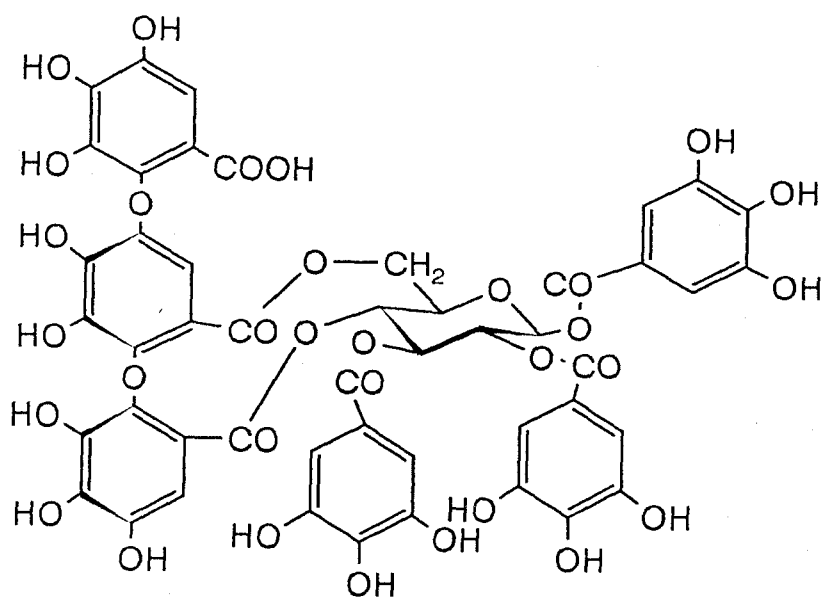
rugosin A (77) [77]
