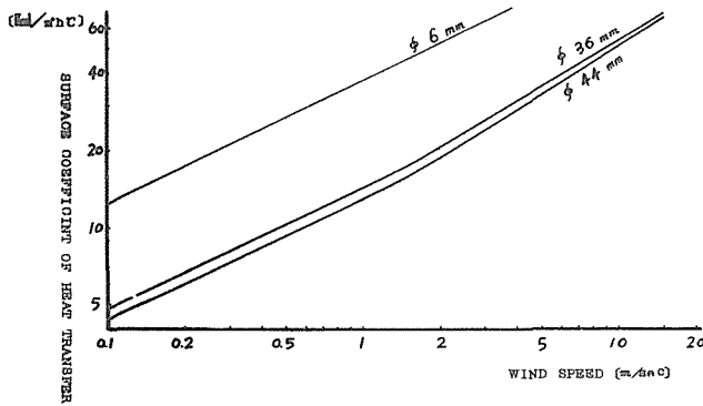
Fig. 3, 対流熱伝達率 \alpha_o と風速との関係
