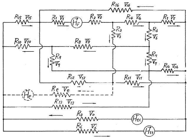
図 - 2 通 気 回 路
