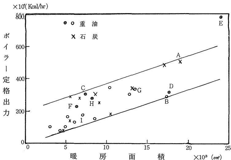
図一 1 暖房面積とボイラー容量の関係
