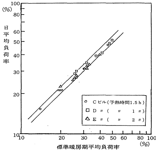
図一五 標準暖房期と1日の平均負荷率の関係
