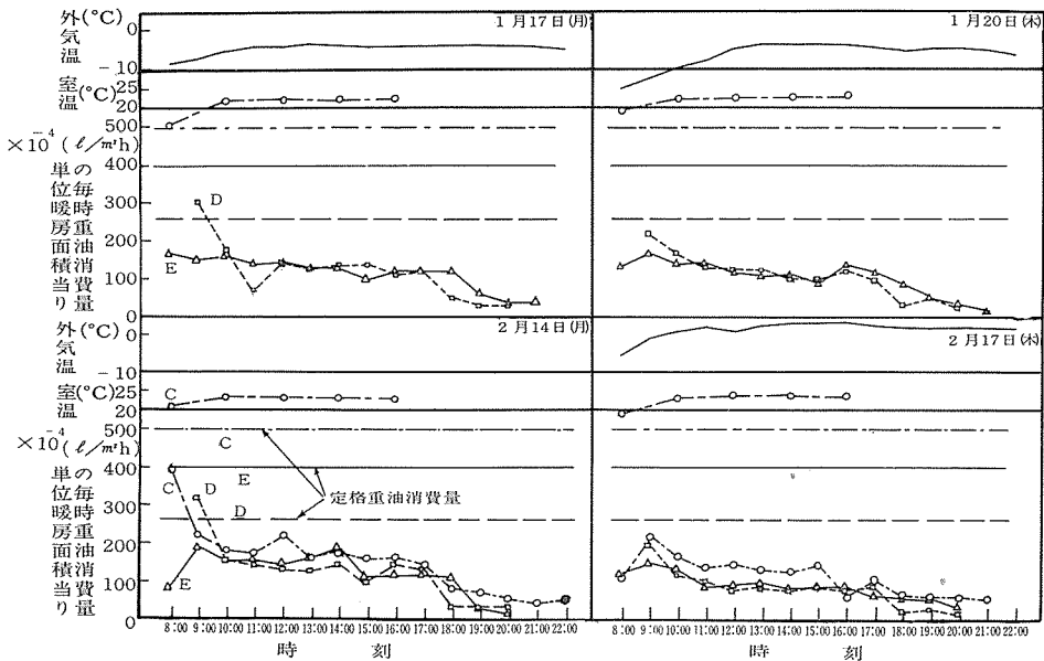
図 4 時刻別重油消費量
