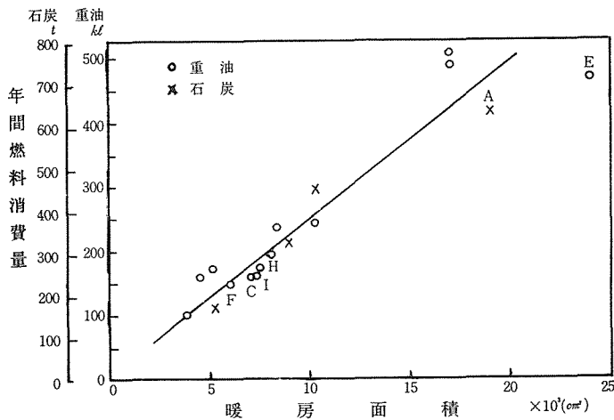
図一2 暖房面積と年間燃料消費量の関係
