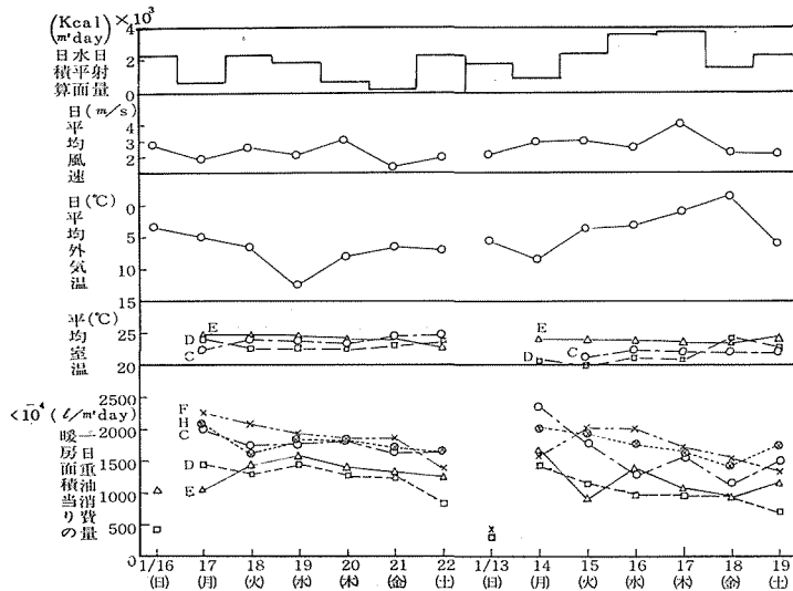
図 3 曜日別重油消費量
