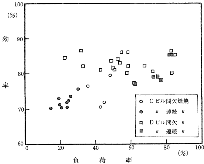
図一 7 負荷率と効率の関係
