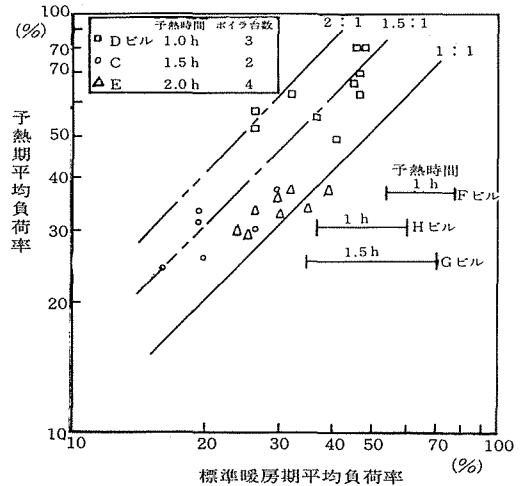
図一六 標準暖房期と予熱期の平均負荷率の関係
