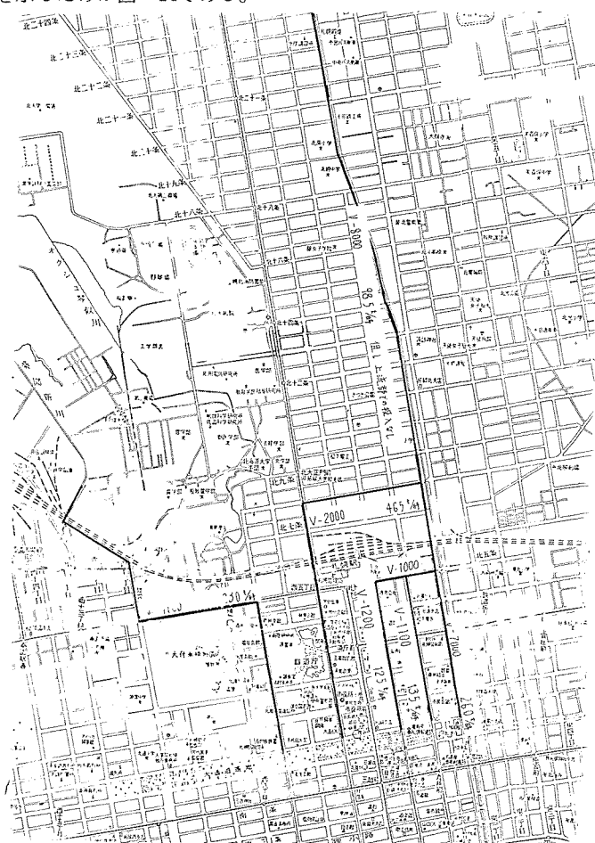
図-14 雪投入可能下水幹線と投入可能量
