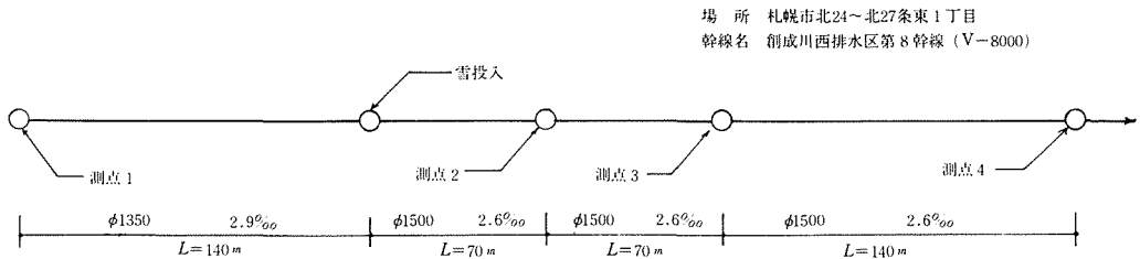
図－3 実験番号 6 実施下水管渠図および測点配置図
