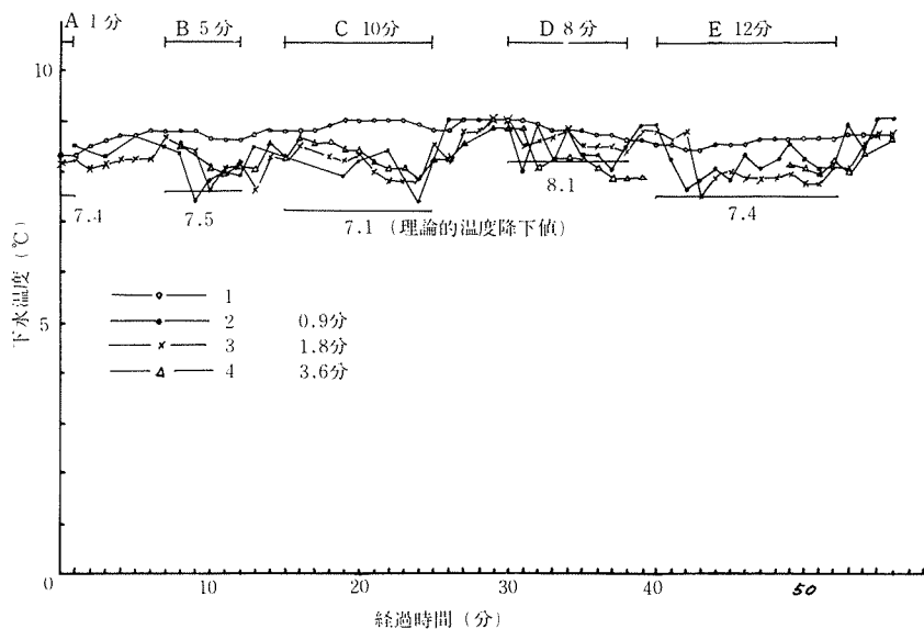
図一10 実験番号 6
