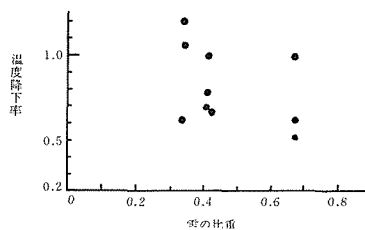
図-12 雪の比重と温度降下率
