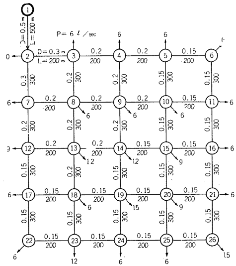
図-7 管網図 (I, II) (流速係数はすべて C=100 )
