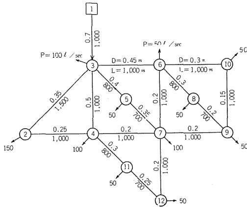
図-6 管網図 (流速係数はすべて C=100 )
