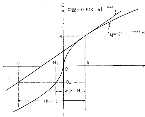
図-1 Q - H 曲線
