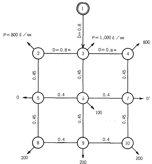
図-8 管網図 (III) (管路長はすべて L=1000\text{m} 、 流速係数はすべて C=100 )
