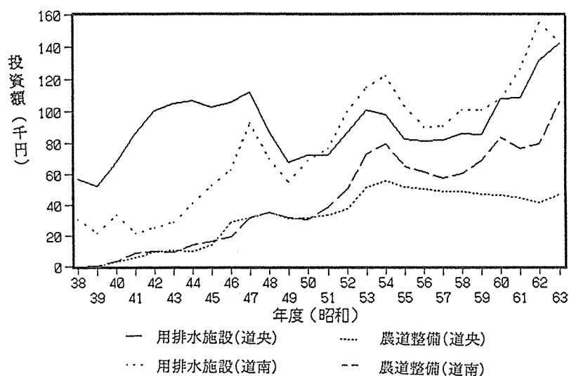
図 2 - A 耕地ha当り農業土地基盤整備事業投資額の推移 (1)
