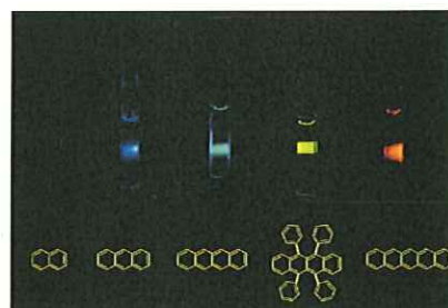
図 2、左からナフタレン、アントラセン、テトラセン、ルブレン、ペンタセンの蛍光。
