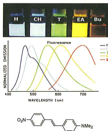
図 3、DNS 蛍光の溶媒効果
