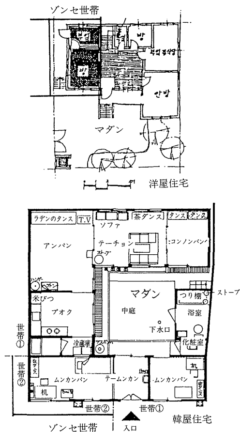
図-2 韓国における現代都市住宅の平面構成 13,14)
