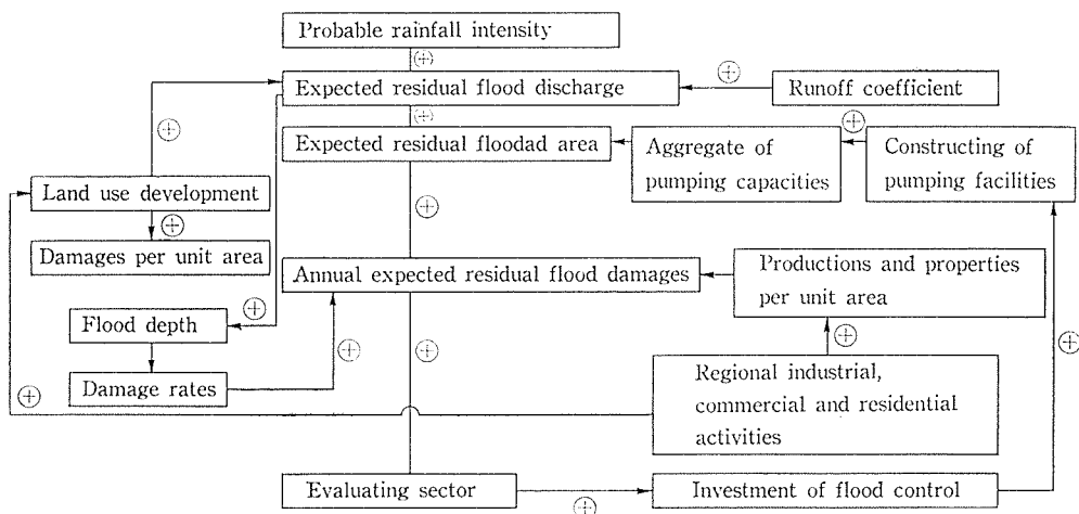
Fig. 2. Flowdiagram of MODEL-I.
