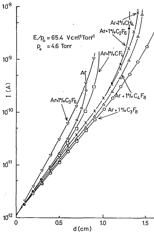
図2 混合ガスの電離電流増倍曲線
