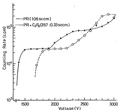
図5 電圧—計数率特性。実線：PRガス，点線：PRガス+ \text{C}_2\text{F}_6 混合ガス
