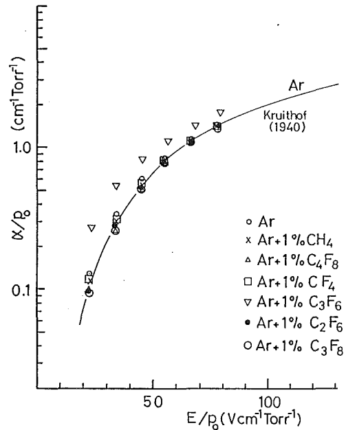
図3 混合ガスの電離係数 \alpha/p ( 20 < E/p < 80 \text{ V/cm Torr} )
