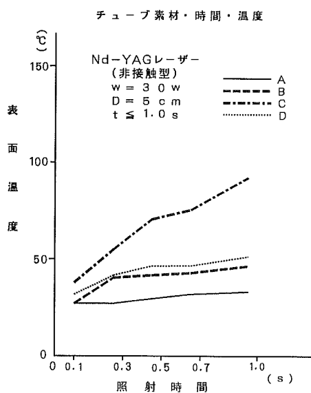
図8 レーザー照射とチューブ表面温度
