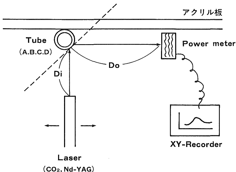
図2 レーザー反射光測定方法
