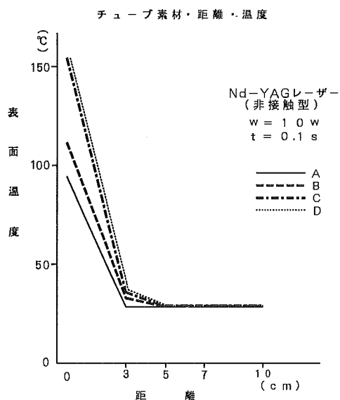
図5 レーザー照射とチューブ表面温度
