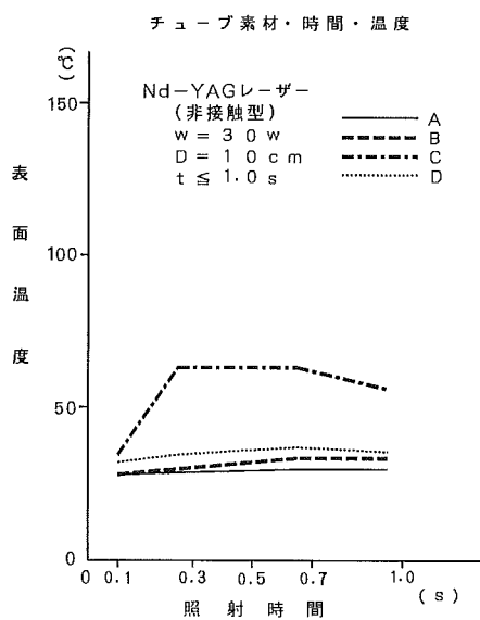
図10 レーザー照射とチューブ表面温度
