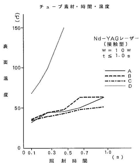
図4 レーザー照射とチューブ表面温度
