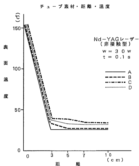
図6 レーザー照射とチューブ表面温度
