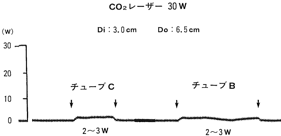
図11 検出した反射曲線例
