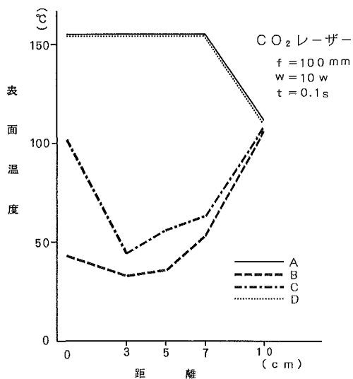
図3 レーザー照射とチューブ表面温度
