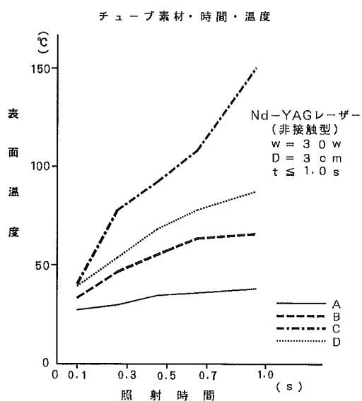
図7 レーザー照射とチューブ表面温度
