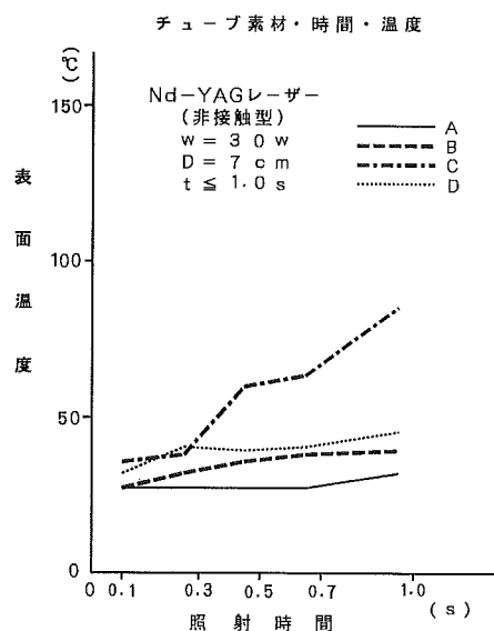
図9 レーザー照射とチューブ表面温度
