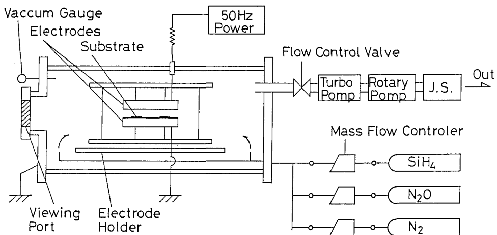
図1 50 Hz プラズマCVD装置全系
