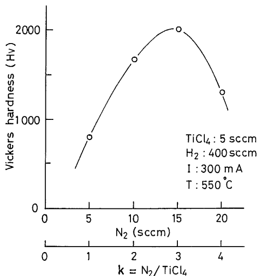
図7 N_2 の流量とヴィッカース硬度計
