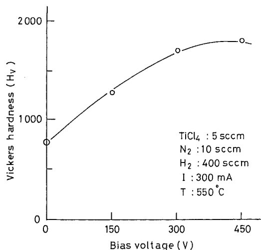
図8 基板バイアス電圧とヴィッカース硬度計
