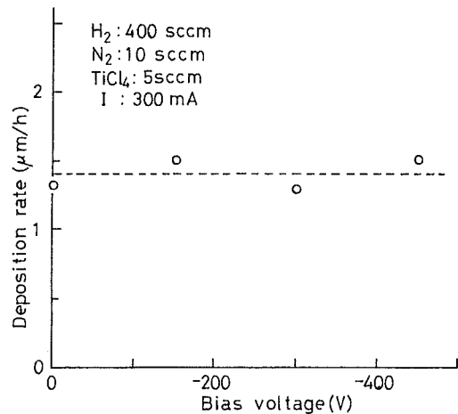
図6 基板バイアス電圧と堆積率
