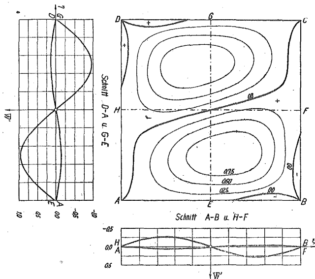
Abb. 17. Schichtlinien der Fläche \tilde{w}' = \tilde{w}'_a + \kappa \tilde{w}'_b für die dritte Familie der dritten Schwingungsart.
