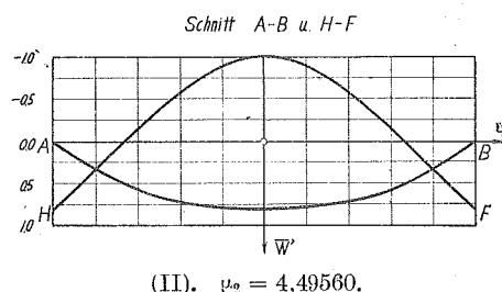
Abb. 5. Schichtlinien der \bar{w}' -Fläche für die erste Familie der ersten Schwingungsart.
