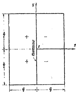
Abb. 13. wb' -Fläche.
