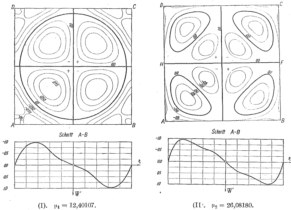
Abb. 9. Schichtlinien der \bar{w}' -Fläche für die erste Familie der zweiten Schwingungsart.
