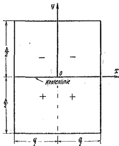
Abb. 12. w'_a -Fläche.
