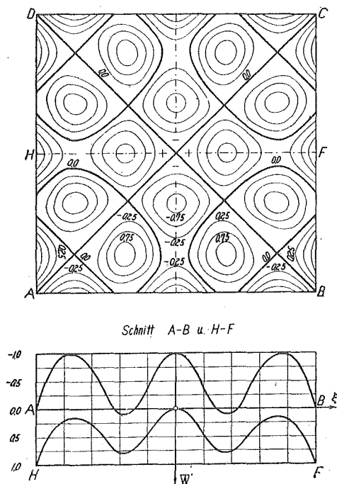
Abb. 21. Schichtlinien der \bar{w}' -Fläche für die zweite Familie der ersten Schwingungsart.
