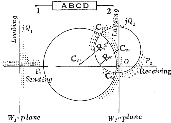
Fig. 2. Transformation of W_1 -plane on W_2 -plane.
