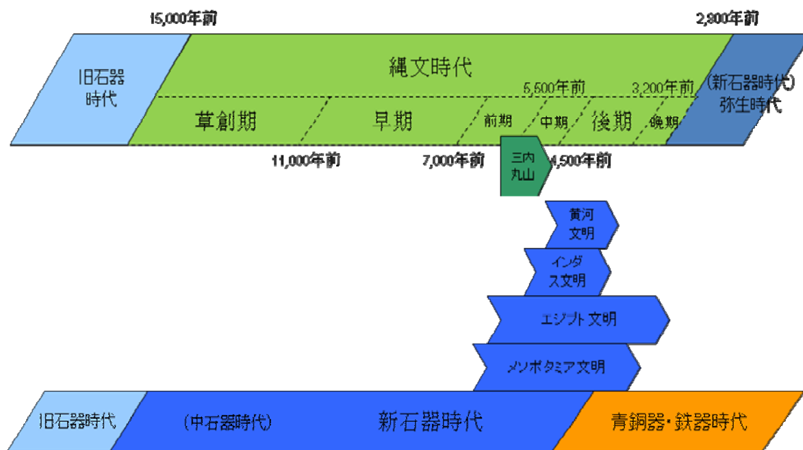
図1-1 縄文時代の区分と四大河文明
