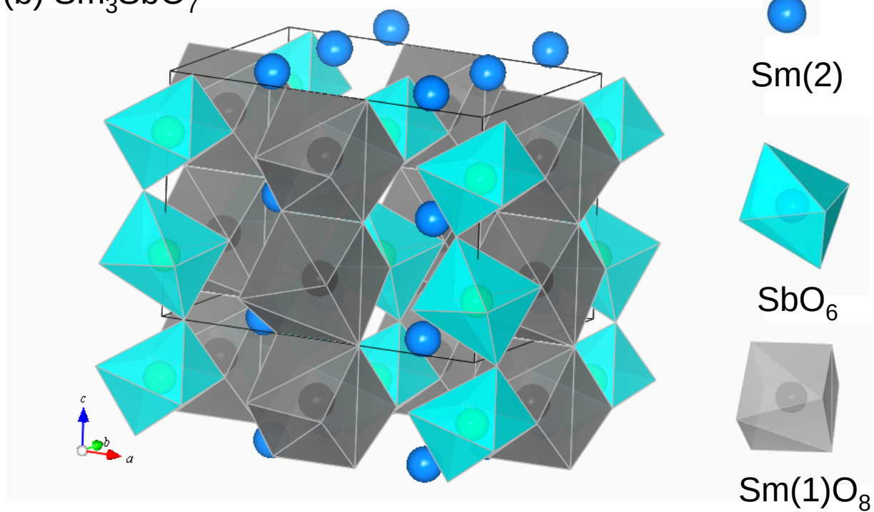
(b) \text{Sm}_3\text{SbO}_7
