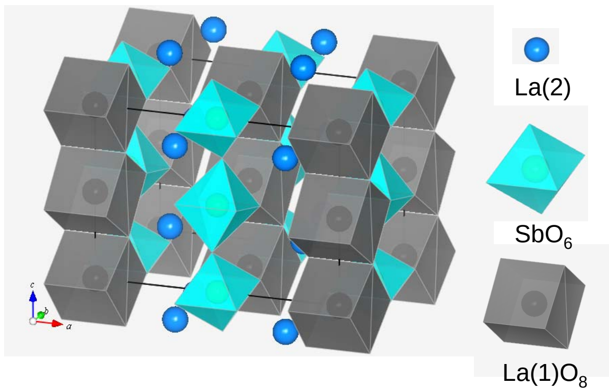
(a) \text{La}_3\text{SbO}_7
