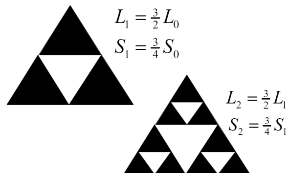
図 42: 正三角形の中央部分から逆正三角形を「なか抜き」していくプロセスでもガスケットは描ける。 S_0, S_1, S_2 は各ステップでの図形の総面積。 L_0, L_1, L_2 は各ステップでの図形の全周囲長。
