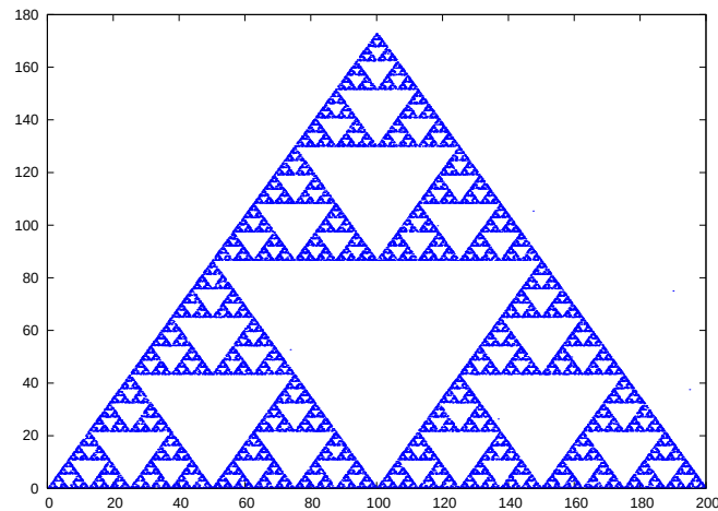
図 41: シェルピンスキー・ガスケット.
