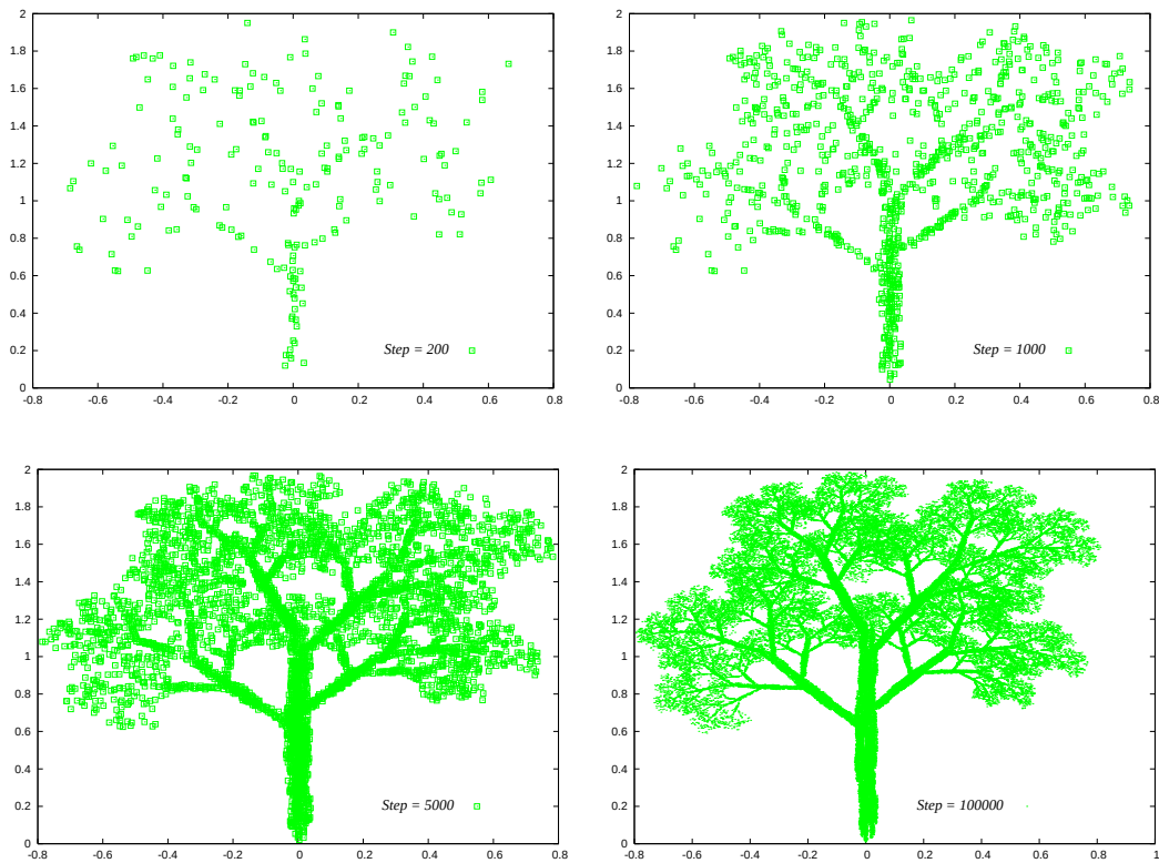
図 40: 計算機を用いて描かれた木. ブロコリに見えなくもない.
