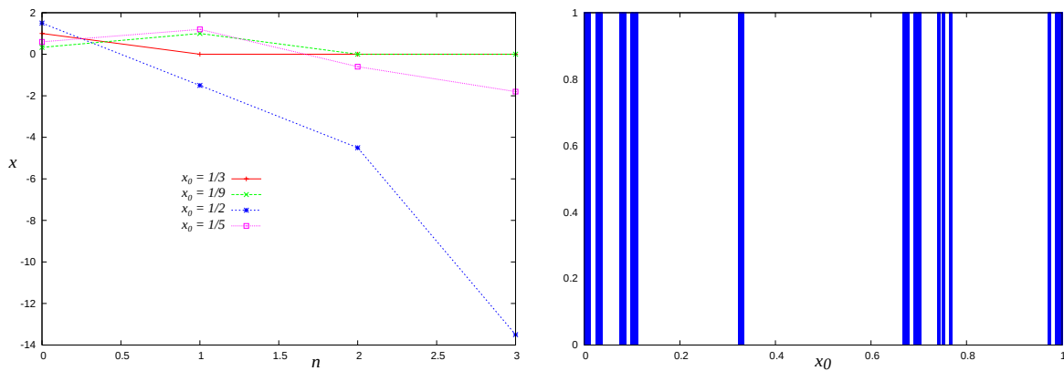
図 44: 写像力学系のゼロへ収束する初期値の集合がコントロール集合を与える例. 左図はいくつかの初期値に対する写像 (197) の数ステップの様子. 右図はゼロに収束する初期値の集合 (図では見やすいように「バーコード」で描いている). これはコントロール集合となる.
