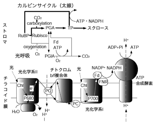
図1：光合成・光呼吸の模式図 9) チラコイド反応において、実線は電子の、点線はエネルギー(光エネルギーまたは励起エネルギー)、破線はプロトン(H + )の移動を示す。
