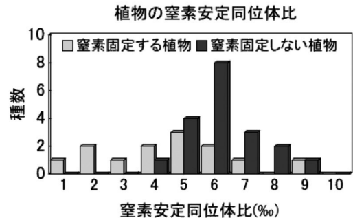
図 6：窒素固定を行なう植物と行なわない植物における窒素安定同位体比 2) 。
