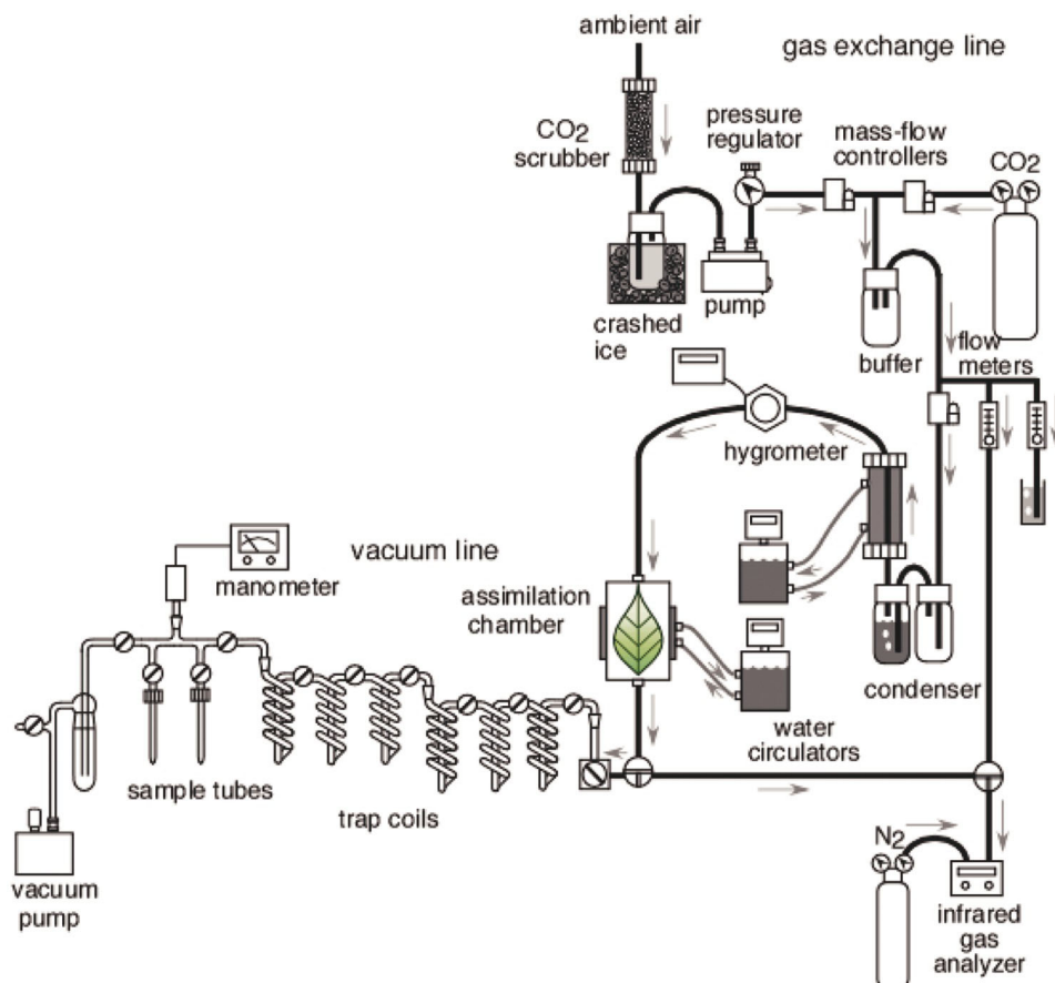
図5：葉内 \text{CO}_2 コンダクタンスを測定するための装置の概略。右側がガス交換測定装置，左側が真空ライン。
