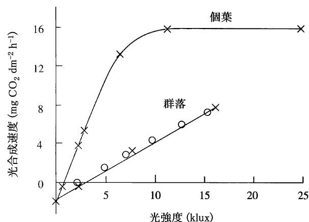
図1：シロガラシの個葉の光—光合成関係と、群落の光—光合成関係（×）。○は M. Monsi と T. Saeki 2) の群落光合成モデルによる推定値を示す。P. Boyesen Jensen 1) を改変。
