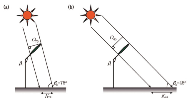
図 5：太陽の入射方向から見た葉の投影面積 ( O ) と、太陽高度 (入射角; \beta_s )、葉の傾斜角 ( \beta_i )、吸収係数 ( K ) の関係の模式図。例として、 \beta_s が 75^\circ (a) と 45^\circ (b) の場合を示す。
