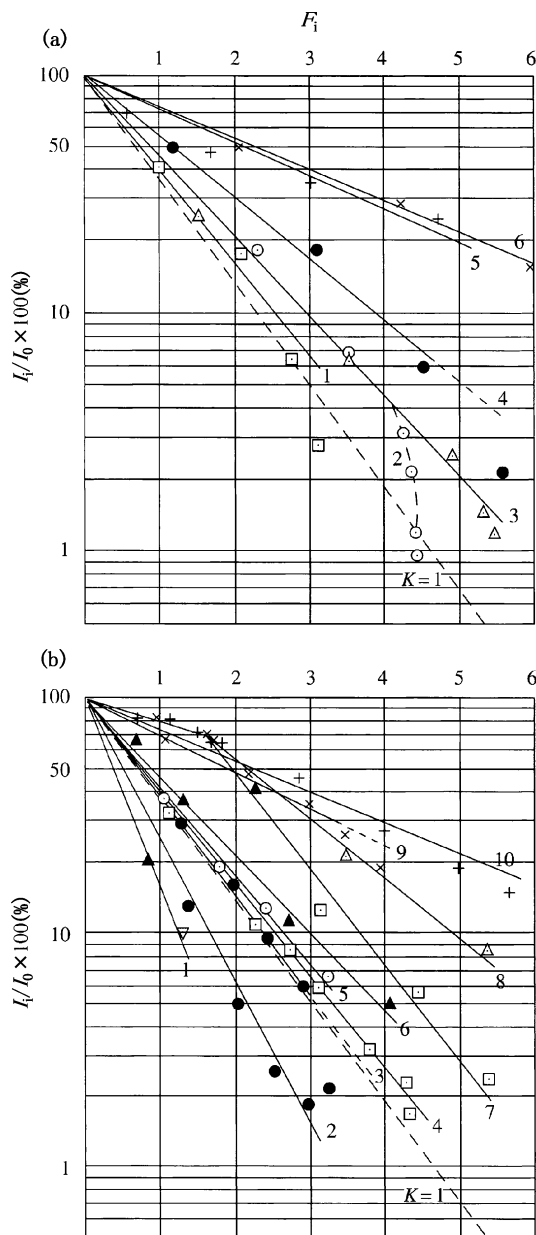
図3：(a)霧ヶ峰山地草原の群落における、相対照度 ( I_i/I_0 \times 100 ) と積算葉面積指数 ( F_i ) の関係。回帰直線の傾きが吸光係数 ( K ) を示す。直線に付記された数字は、種を示している。1：ミヤコザサ・ワラビ群落 (1949年9月15日)、2：ミヤコザサ群落 (1951年8月29日)、3：ミヤコザサ群落 (1949年9月14日)、4：ミヤコザサ群落 (1949年8月7日)、5：ススキ群落 (1949年9月15日)、6：ススキ群落 (1949年7月6日)。(b) 1：キカラスウリ群落 (1949年9月30日)、2：フキ群落 (1950年4月28日)、3：アカザ群落 (1949年6月28日)、4：ノウルシ群落 (1951年5月5日)、5：クイモ群落 (1949年5月26日)、6：キャラボク群落 (1949年6月13日)、7：オギ・ノウルシ群落 (1950年4月30日)、8：ヨシ・ナガボノシロワレモコウ群落 (1949年6月3日)、9：オギ群落 (1949年6月15日)、10：ヨシ・ノカラムツ群落 (1949年7月27日)。M. Monsi と T. Saeki 2) を改変。
