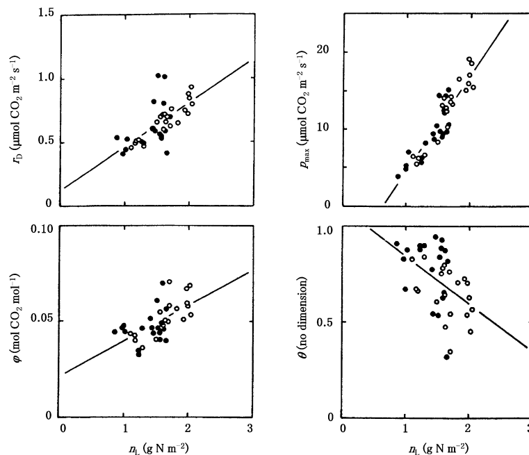
図4：セイタカアワダチソウ群落における、単位葉面積あたりの窒素含量 ( n_L ) と飽和光下光合成速度 ( p_{\text{max}} )、光—光合成曲線の初期勾配 ( \varphi )、曲度 ( \theta )、暗呼吸速度 ( r_D ) の関係。●は高密度、○は低密度群落の、様々な層から採取した葉を示す。T. Hirose と M. J. A. Werger 12) を改変。
