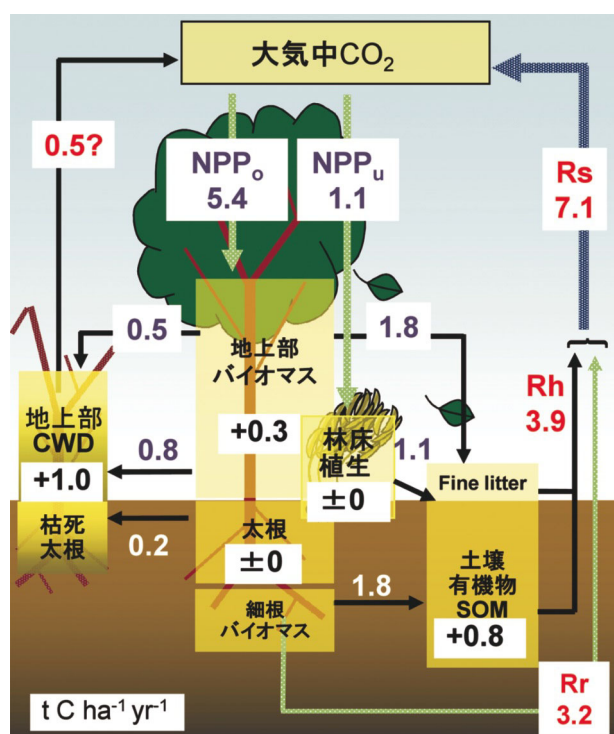
図 6：高山サイトでの炭素循環のコンパートメントモデル。□は生態系内の炭素プールを示し、1 年間の収支を数値で示している (1999 年から 2003 年までの 5 年間の平均値)。矢印は各プール間の炭素フラックスを示し、1 ha 当たりでの 1 年間の移動量を示している。
