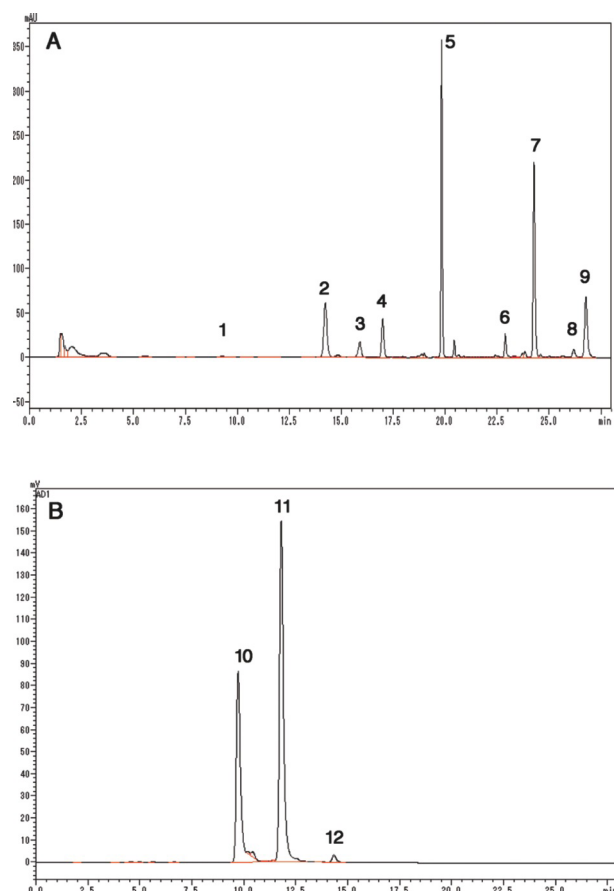
図4：Zapataらの系による光合成色素の分離 A. シロイヌナズナの葉の抽出液の分離。横軸は溶出時間(分)、縦軸は410 nmにおける吸収。：1.chlorophyllide a , 2. pheophorbide a , 3.neoxanthin, 4.violaxanthin, 5.lutein, 6.chlorophyll b , 7.chlorophyll a , 8.pheophytin a , 9.β-carotene B. クロロフィル代謝中間体(標準物質)の分離。蛍光検出器(Shimadzu, RF550)を用いて、励起波長417 nm, 蛍光波長600 nmで測定した。：10.Mg-protoporphyrin IX, 11.Mg-protoporphyrin IX monomethylester, 12.protoporphyrin IX
