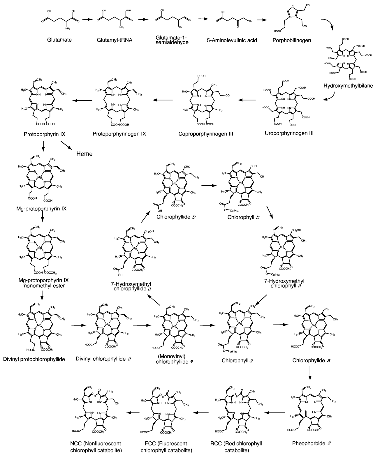
図3：被子植物のクロロフィル代謝経路
