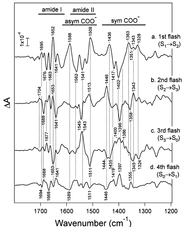
図 4：光化学系 II における酸素発生 S 状態サイクルの閃光誘起 FTIR 差スペクトル。1 (a), 2 (b), 3 (c), 4 (d) 閃光目のスペクトルは、それぞれ S 状態サイクルの \text{S}_1\rightarrow\text{S}_2 , \text{S}_2\rightarrow\text{S}_3 , \text{S}_3\rightarrow\text{S}_0 , \text{S}_0\rightarrow\text{S}_1 遷移の際の構造変化を示す。試料は好熱性シアノバクテリア T. elongatus より調製した光化学系 II コア蛋白質複合体の水和試料。電子受容体としてフェリシアン化物イオンを含む。温度は 10^\circ\text{C} 。
