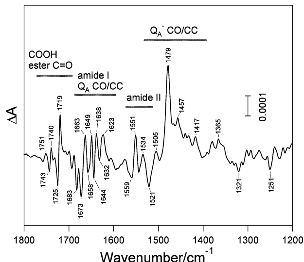
図 3: 光化学系 II における第一キノン電子受容体 \text{Q}_\text{A} の一電子還元による光誘起 FTIR 差スペクトル。試料はハウレンソウより調製した光化学系 II 膜標品。電子供与体として \text{NH}_2\text{OH} , 電子伝達阻害剤として DCMU を含む。温度は 250 K。
