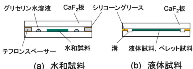
図 2: FTIR 差スペクトル測定用試料セルの例。(a) 水和試料; (b) 液体またはペレット試料。
