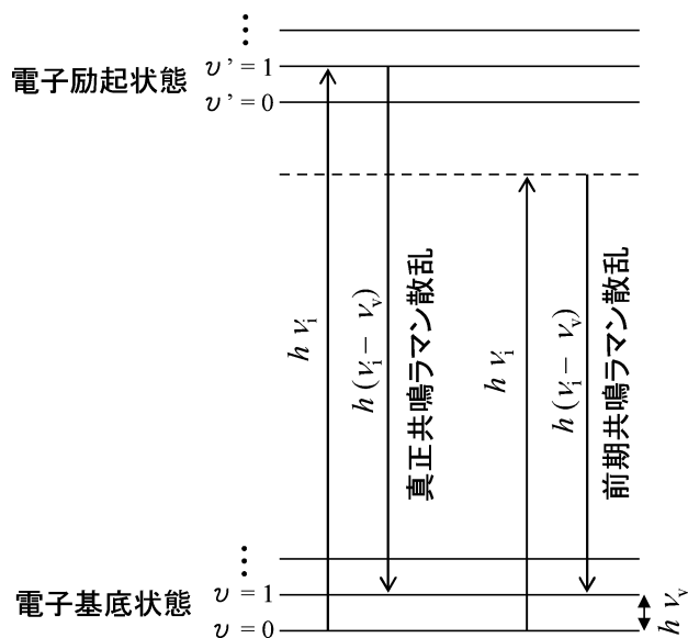
図1：真正共鳴ラマン散乱と前期共鳴ラマン散乱。
