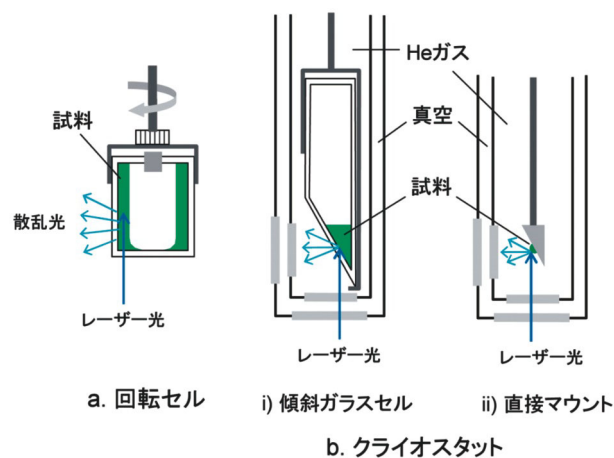
図2：光合成試料に適したラマン散乱測定を試料部。(a) 液体試料用回転セル。(b) クライオスタットによる試料凍結；(i) 傾斜石英ガラスセル，(ii) 直接マウント試料。
