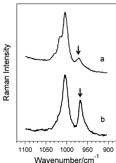
図4：紅色光合成細菌のクロマトフォアにおけるカロテノイドの共鳴ラマンスペクトル（CH面外変角振動領域）。（a） Rhodobacter sphaeroides （b） Chromatium vinosum 。CH面外変角振動バンドを矢印で示す。 Rb. sphaeroides の弱いCH面外変角振動バンド、及び Ch. vinosum の強いCH面外変角振動バンドは、それぞれ、ポリエチレン鎖の平面、及び捩れ構造を表す。
