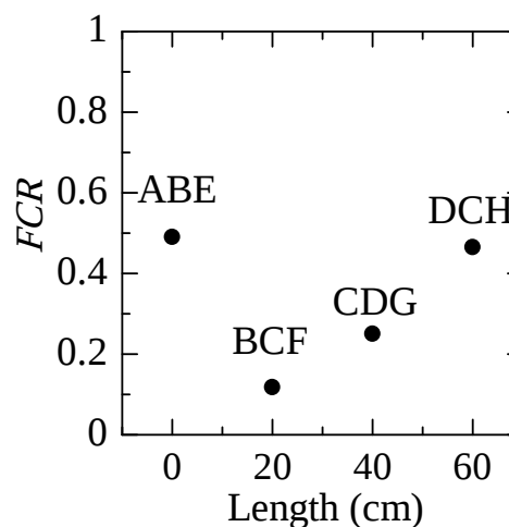
図7 亀裂密着度
