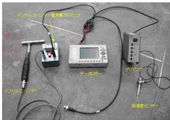
図 1 計測機器
