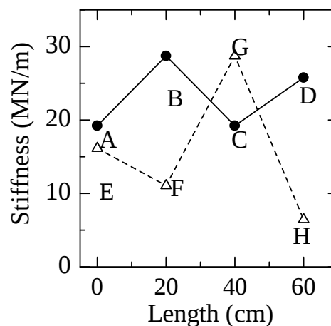
図6 バネ係数
