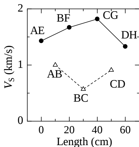
図5 弾性波速度
