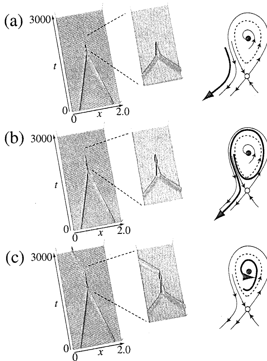
図 4: (a)対消滅 ( D_v = 2.9450 \times 10^{-4} ). (b) 振動した後消滅 ( D_v = 2.9465 \times 10^{-4} ). (c) 融合 ( D_v = 2.9480 \times 10^{-4} ). 右図はそれぞれに対応した融合後の模式的な解の流れ. (図 3(b)C 参照)
