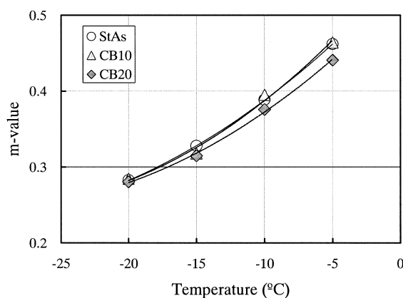
b) m-value
