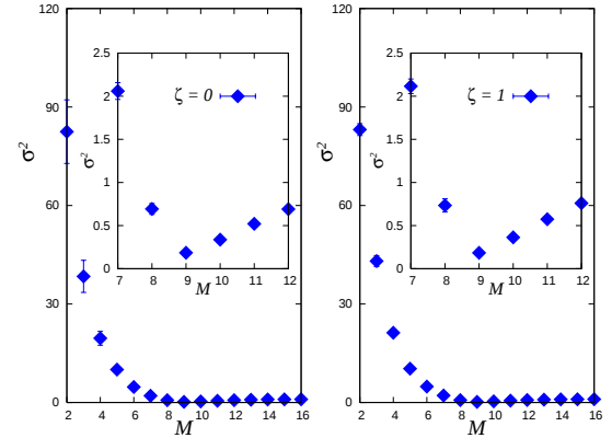
Fig. 6 ボラティリティの履歴数 M 依存性. 左図は真市場履歴 ( \zeta = 0 ), 右図は偽市場履歴 ( \zeta = 1 ) の場合. 挿入図は図の 7 \leq M \leq 12 の領域を拡大したものである. これらの挿入図より, ボラティリティの非単調性が確認できる (この場合, どちらも M = 9 ). N = 2^{10} + 1 = 1025 , 図中の誤差棒は 10 回の独立試行に基づき算出した.
