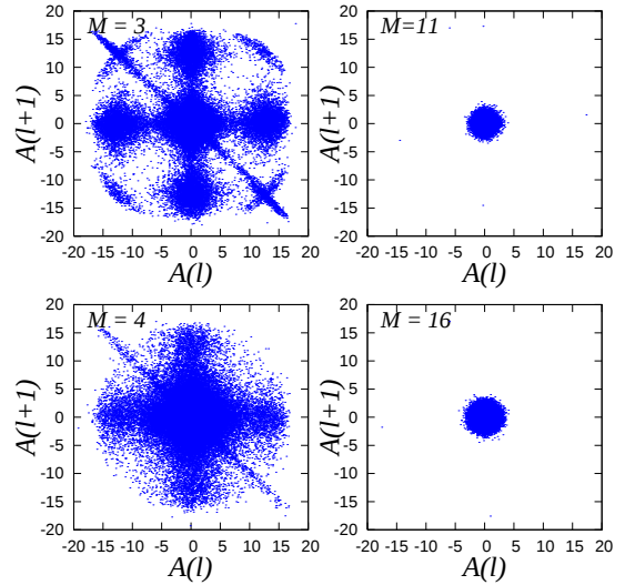
Fig. 3 総入札価格の連続する 2 ラウンド間の値: A(l) と A(l+1) のプロット. それぞれ、 M = 3 ( P = 2^3 = 8 ), M = 4 ( P = 2^4 = 16 ), M = 11 ( P = 2^{11} = 2048 ), M = 16 ( P = 2^{16} = 65536 ). \zeta = 1 の偽市場履歴の場合. システムサイズは N = 2^{10} + 1 = 1025 .
