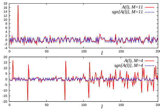
Fig. 2 総入札価格 A(l) , および、その符号 \text{sgn}[A(l)] の時間変化. 下図は M = 4 ( P = 16 ), 上図は M = 11 ( P = 2048 ). システムサイズは N = 2^{10} + 1 = 1025 . 真市場履歴 \zeta = 0 の場合. この繰り返しゲームの各ラウンドにおいて、各トレーダが情報ベクトルとして共有する市場のマクロ情報は破線で与えられる。
