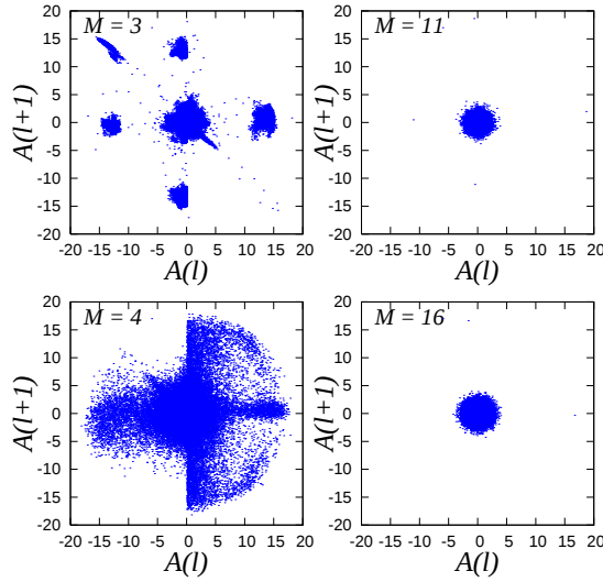
Fig. 4 総入札価格の連続する2ラウンド間の値: A(l) と A(l+1) のプロット. それぞれ, M = 3 ( P = 2^3 = 8 ), M = 4 ( P = 2^4 = 16 ), M = 11 ( P = 2^{11} = 2048 ), M = 16 ( P = 2^{16} = 65536 ). \zeta = 0 の真市場履歴の場合. システムサイズは N = 2^{10} + 1 = 1025 .
