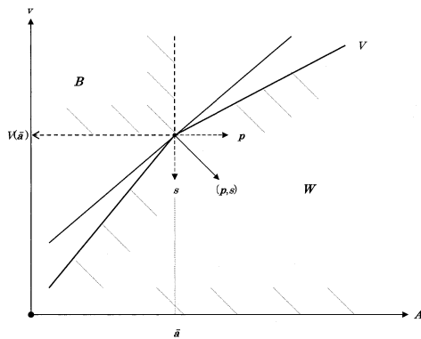
第4-2図： B と W の分離—微分不可能な V のケース
