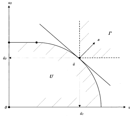
第5図： \Gamma と U の分離
