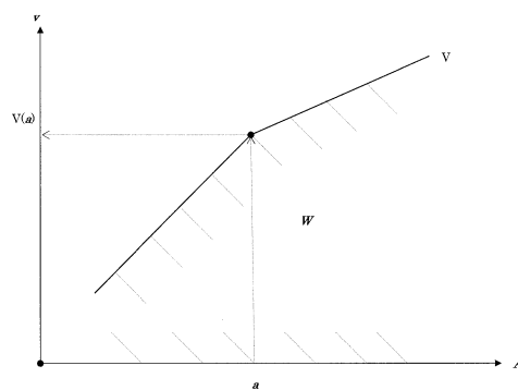
第1-2図：WとVの関係
