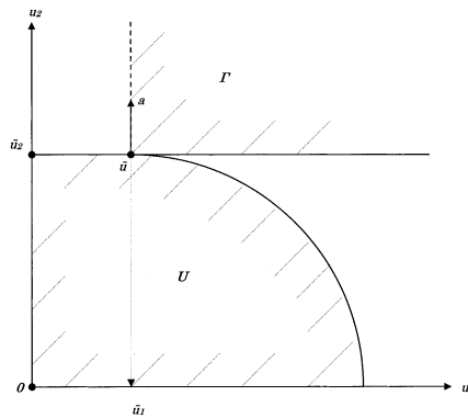
第6図： \mathbf{a} > 0 とならないケース
