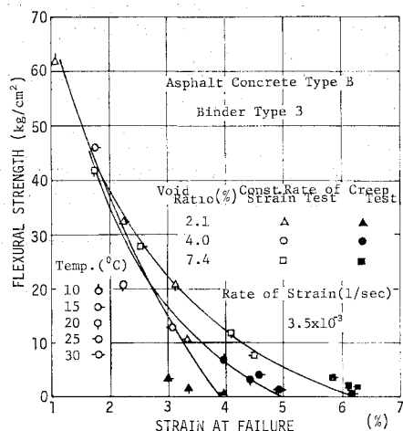
図一 空隙率が破壊包絡線に及ぼす影響
