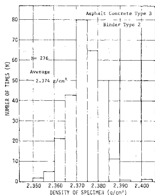
図-1 供試体の密度のヒストグラム
